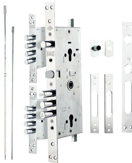
Cerradura de Incrustar Multipunto Kale 256G
